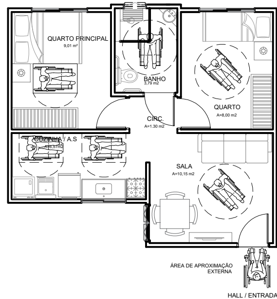
PLANTA BAIXA PAV. TÉRREO UNIDADE ADAPTÁVEL
